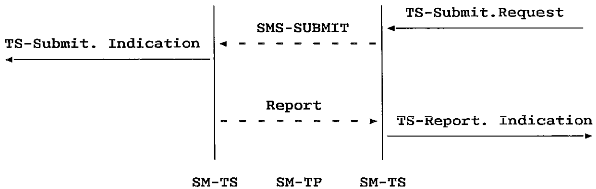
b) The SM MO case
