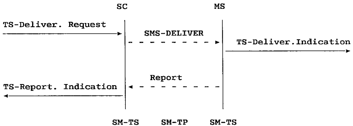
a) The SM MT case
